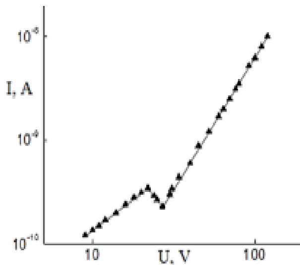
Şək.1. Şüalanmış TlGaS 2 monokristallarının volt-amper xarakteristikası
