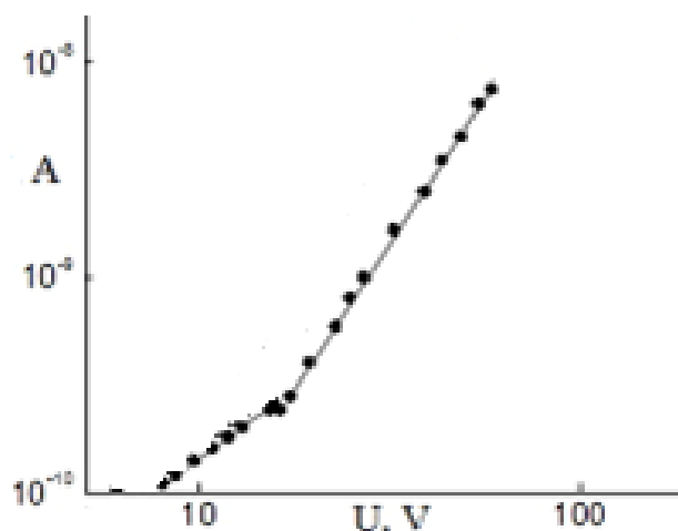
Şək.2. Şüalanmış TlGaSe 2 monokristallarının volt-amper xarakteristikası
