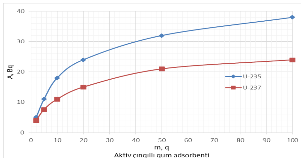
Şək. 2. 100 qram aktiv çinqıllı qum adsorbenti kütləsi ilə 100 ml sulu məhluldan (1500 Bq/l) tutulmuş {}_{92}\text{U}^{235} və {}_{92}\text{U}^{237} izotoplarının miqdarı (qamma spektroskopiyası ilə təyin edilmiş aktivlikləri).
