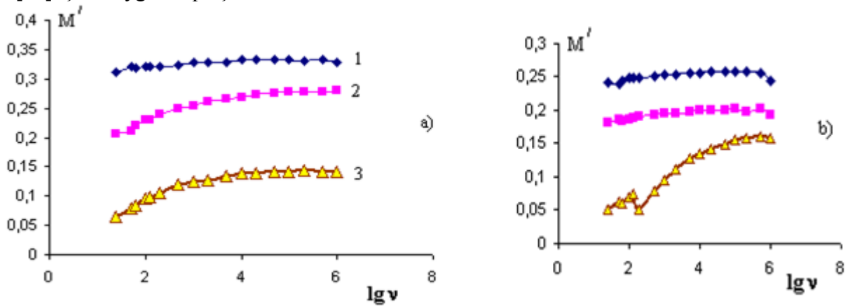
Şək.2. Elektrik modulunun həqiqi hissəsinin \gamma -şüalanmadan əvvəl (a) və sonra (b) tezlikdən asılılığı M'=f(\lg \nu) : a) D=0 , 1- \text{YSPE} + 5\% \text{TiO}_2 , 2- 10\% \text{TiO}_2 ; 3- 20\% \text{TiO}_2 ; b) D=200\text{kQr} , 1- \text{YSPE} + 5\% \text{TiO}_2 , 2- 10\% \text{TiO}_2 ; 3- 20\% \text{TiO}_2 .
