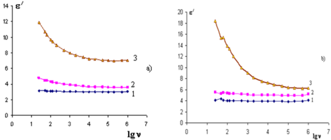
Şək.1. Dielektrik nüfuzluğunun həqiqi hissəsinin \gamma -şüalanmadan əvvəl (a) və sonra (b) tezlikdən asılılığı \epsilon'=f(lg \nu) : a) D=0 , 1-YSPE +5% TiO 2 , 2-10% TiO 2 ; 3-20% TiO 2 ; b) D=200kQr , 1-YSPE +5% TiO 2 , 2-10% TiO 2 ; 3-20% TiO 2 .
